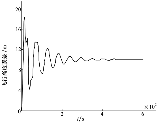
a) 编队飞行垂直误差
