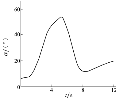
b) 无人机的迎角
