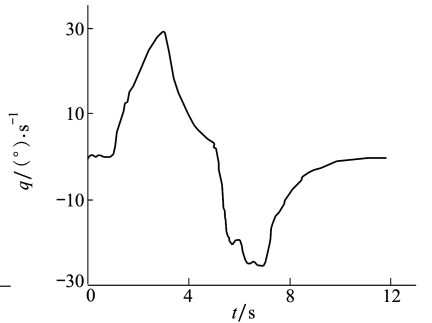
f) 无人机的俯仰角速度
