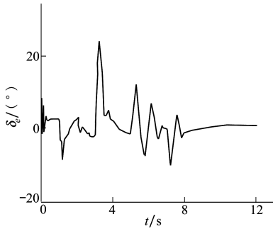
d) 无人机的平尾偏角
