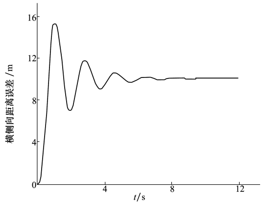
b) 横侧向距离误差
