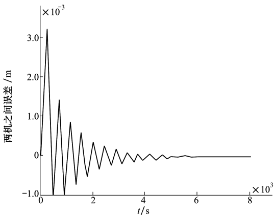
c) 同飞机两机之间的距离
