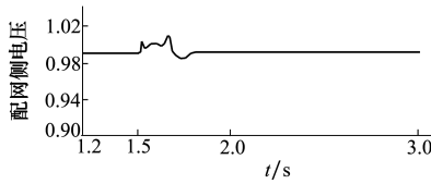
a) 配网侧 PCC 点电压波形
