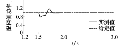
b) 微网侧 PCC 点功率波形
