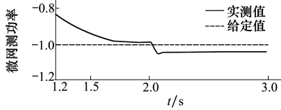
b) 微网侧 PCC 点功率波形
