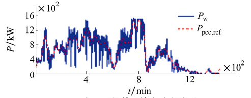
a) 平抑前后输出功率波形
