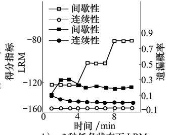
a) 2种任务状态下错误开始和得分指标对比 b) 2种任务状态下LRM和遗漏概率对比
