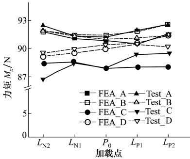
a) 力矩M x -加载点曲线
