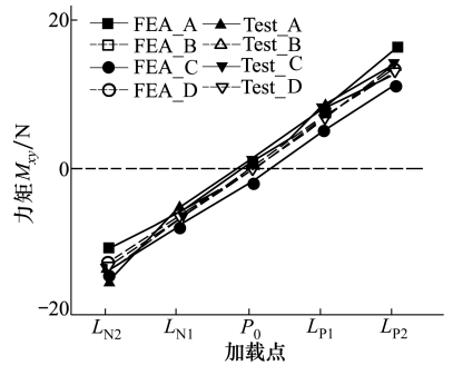
c) 力矩M xy -加载点曲线
