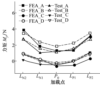
b) 力矩M y -加载点曲线
