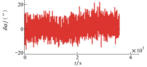
a) 观测值 alpha 的新息序列
