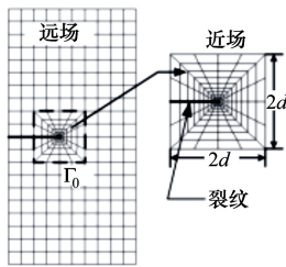
b) 有限元网格
