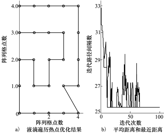
a) 液滴遍历热点优化结果 b) 平均距离和最近距离
