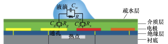
b) 冷却模型及 RC 网络
