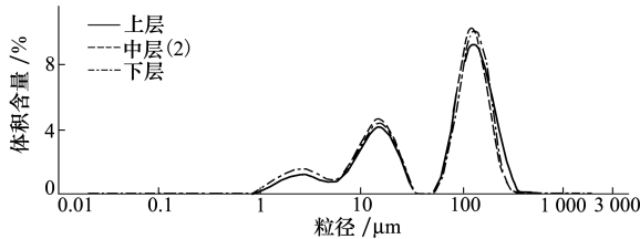
a) 不同高度处铝粉样本测试结果
