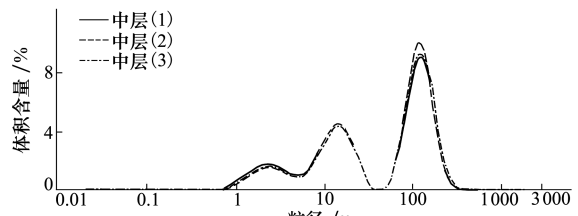
b) 同一高度不同位置处铝粉样本测试结果
