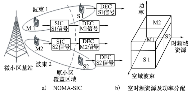
a) NOMA-SIC b) 空时频资源及功率分配
