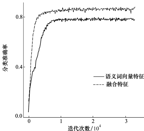
a) 融合特征和语义词向量特征的零样本图像分类
