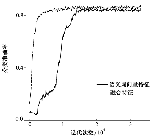
b) 融合特征和语义词属性特征的零样本图像分类
