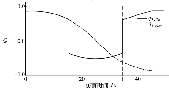
d) q_3 随时间变化
