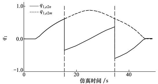
b) q_1 随时间变化
