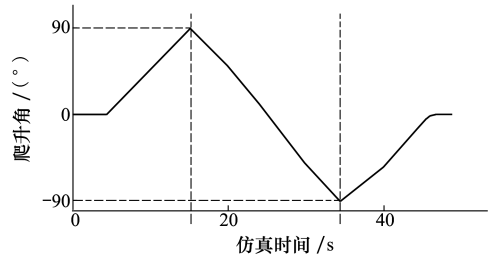
a) 爬升角随时间变化
