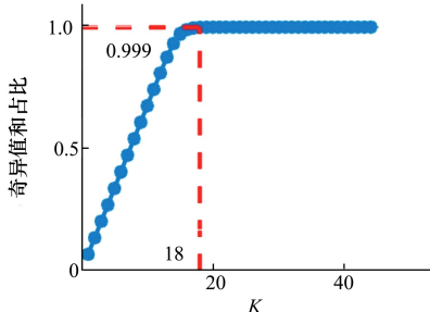
b) 前 K 阶奇异值和占比
